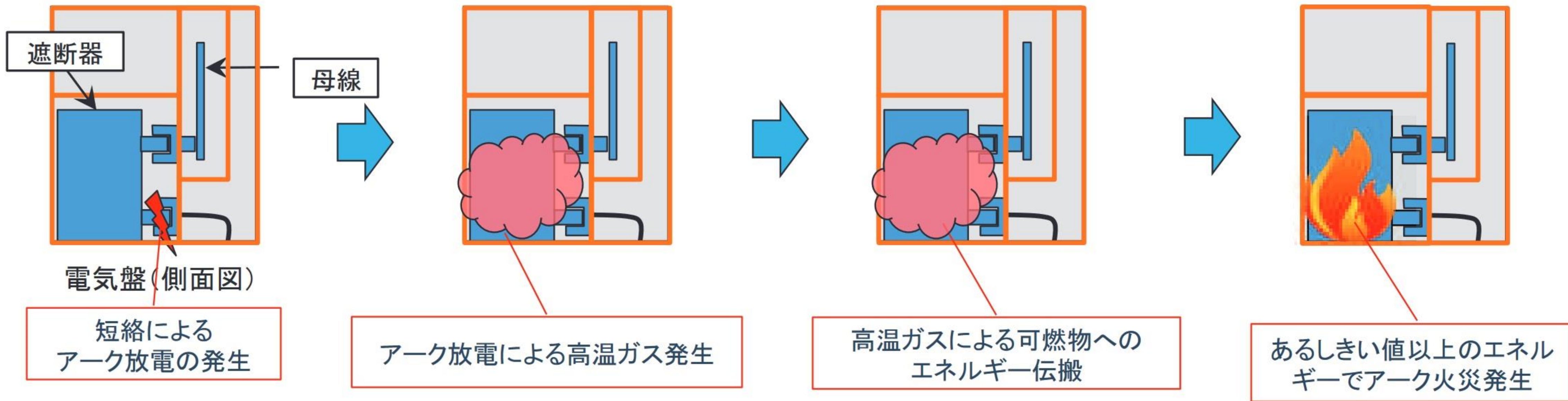
図1 アーク火災発生のメカニズム
