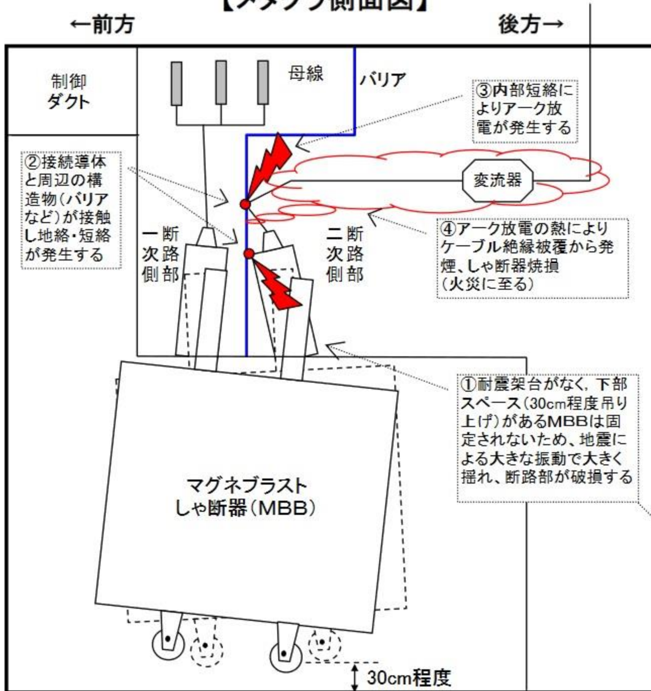
【メタクラ側面図】
