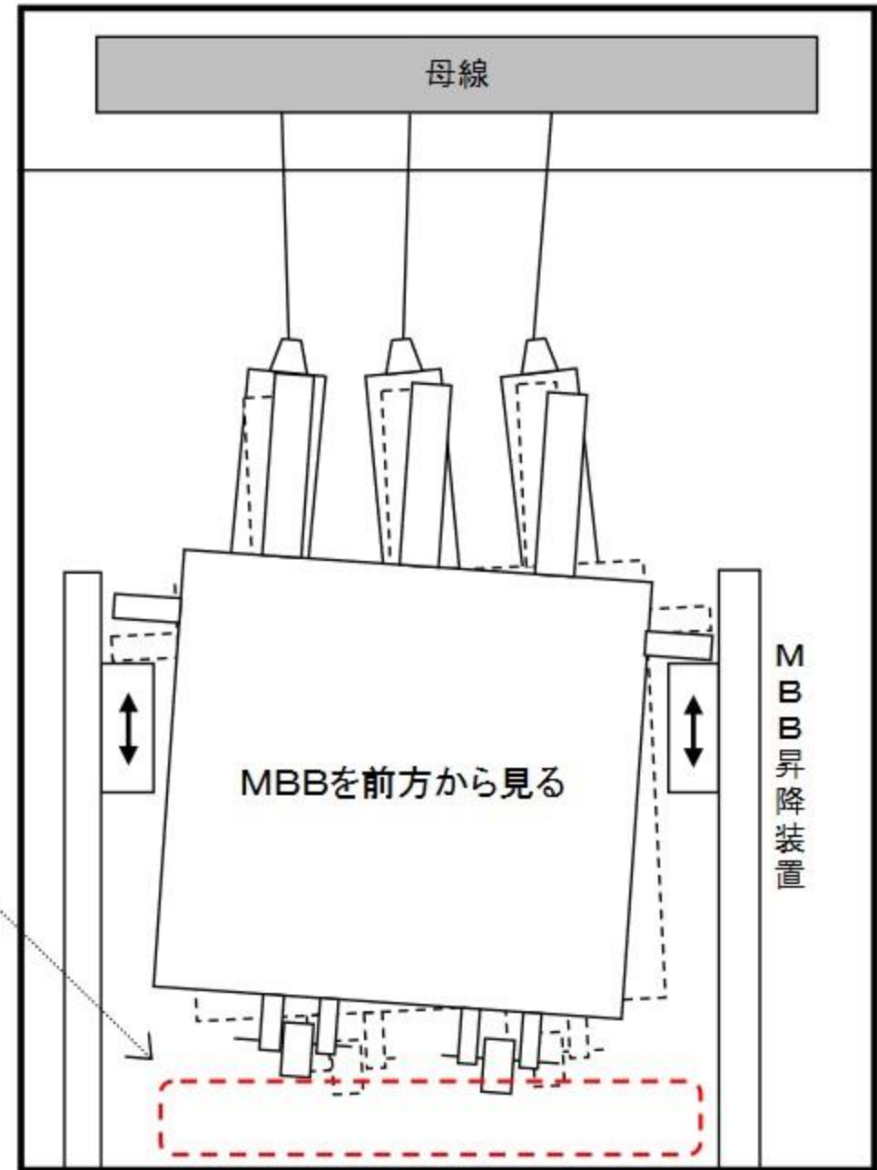
【メタクラ正面図】
